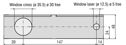
optoNCDT 2310-50BL
